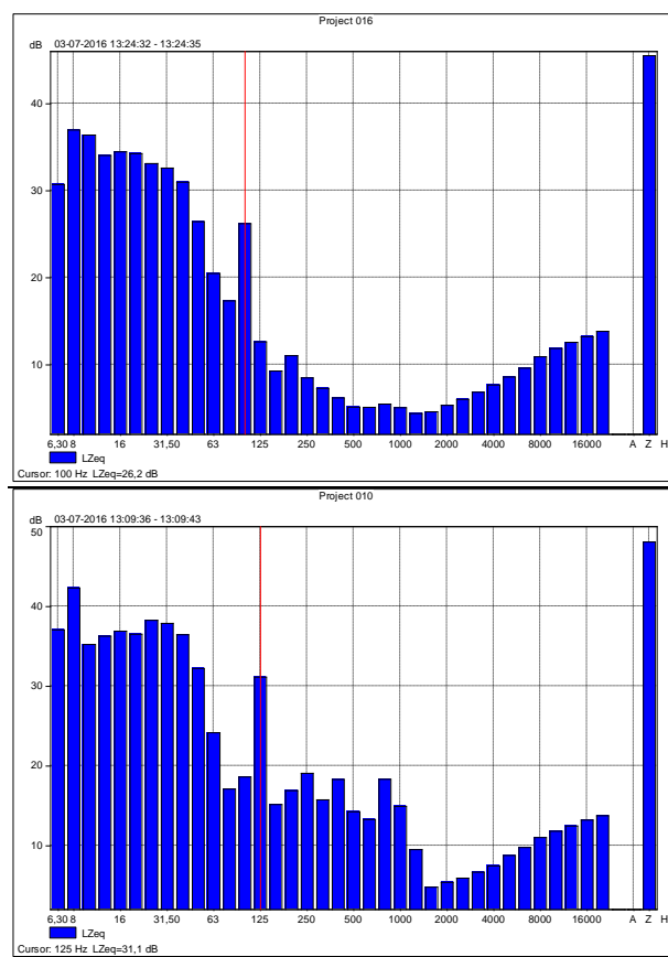
Figuur 2: Nulmeting achtergrondruis van onderzoekruimte (in stilte)
